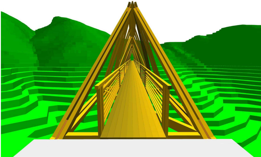
Variante "TOBLERONE"
