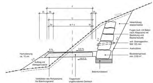
Fig. 15: Blocksteinmauer bzw. Betonmauer
